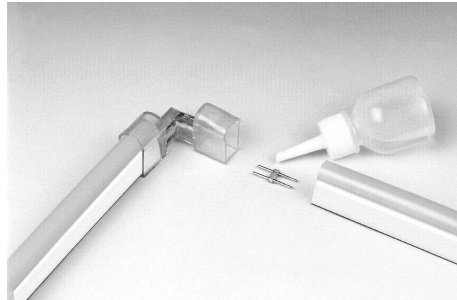
Mit L-Verbindungsstück
